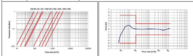
Мал. 2 Графіки залежності відносної похибки лічильників від об'ємної витрати
