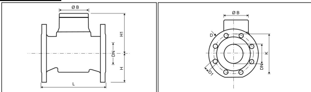
Мал. 1 Лічильник води Wesan
