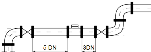
Рис. 4 Схема встановлення лічильника води
