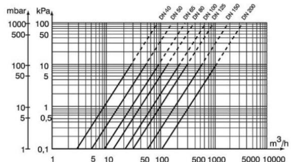
Рис.3 Крива втрати тиску лічильників води типу WI
