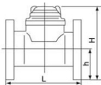
Рис.1 Габаритні розміри лічильників води типу WI
