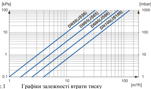
Рис. 1 Графіки залежності втрати тиску лічильників від об'єму витрати
