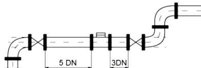
Рис. 4 Схема встановлення лічильника води
